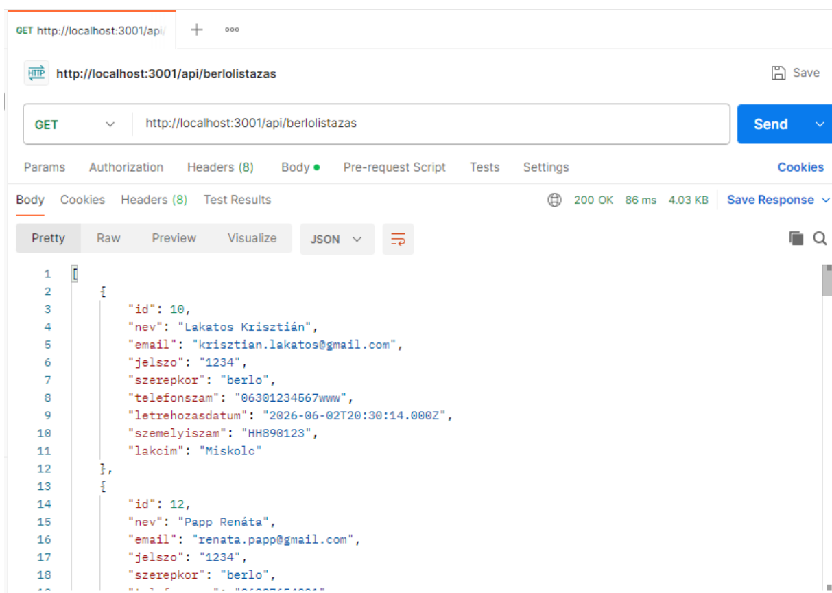
1.Kép: Bérlok listázásának Postman tesztelése.
